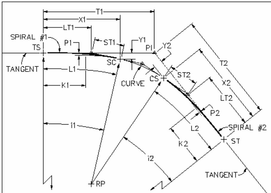
شکل ۴ - ۵ : قوس کلوتویید
