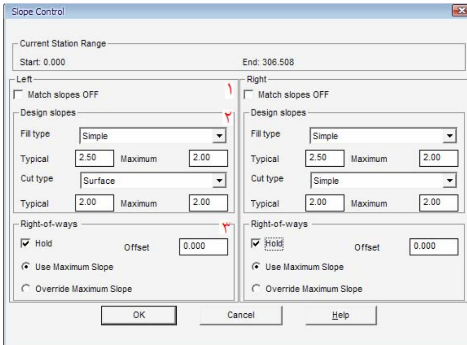
شکل ۶-۸ : پارامترهای شیب شیروانی
