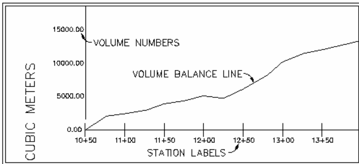
شکل ۲ - ۱۰ : منحنی بروکنر
